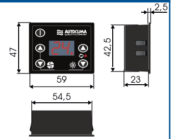
Centralina digitale di controllo Digital control unit Centrale digitale de contrôle Digitale Steuergerät Centralita digital de control
